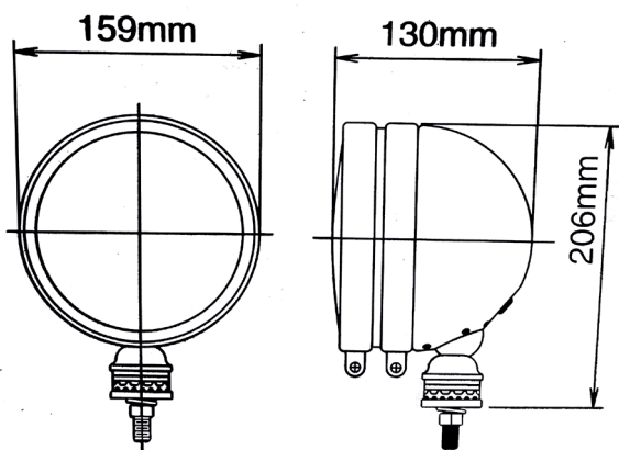
FARO LUNGA PORTATA
